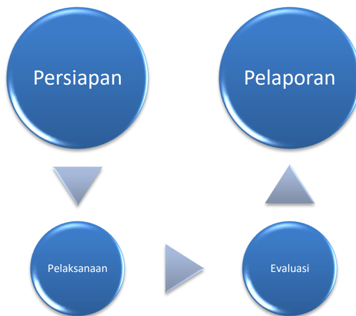
Gambar 1. Alur Pelaksanaan
